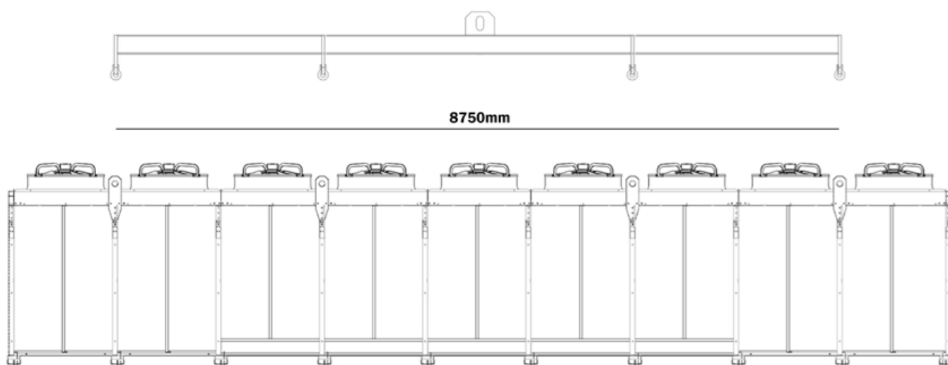
JV 2x9 - Totale 8 punti di sollevamento
