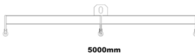
JV 2x4 - Totale 4 punti di sollevamento
