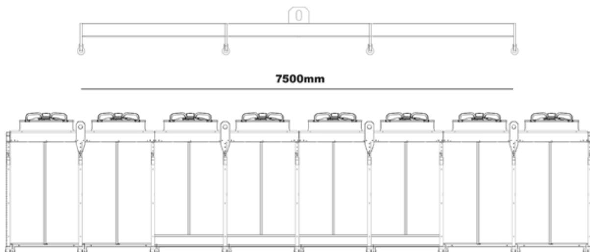
JV 2x8 - Totale 8 punti di sollevamento
