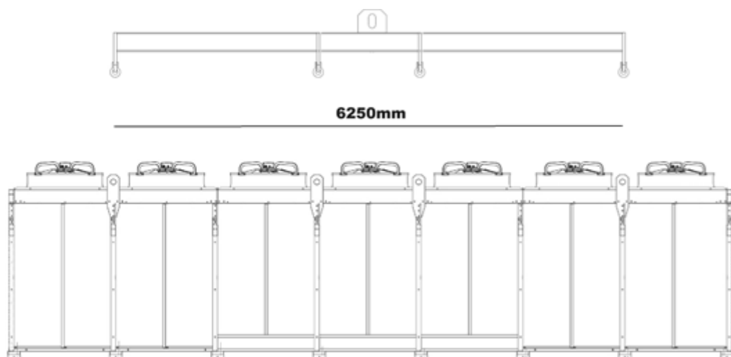
JV 2x7 - Totale 8 punti di sollevamento
